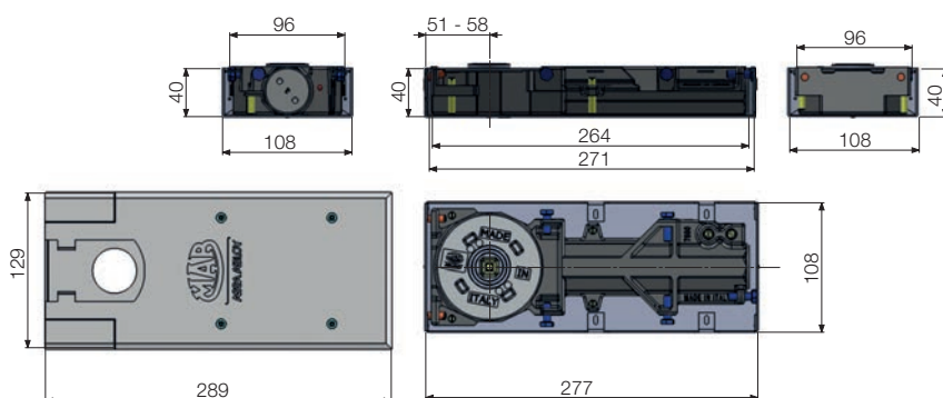
Podni zatvarač
