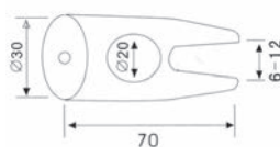
Konektor* staklo-šipka debljina stakla 6/12 mm
