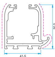
IG OG F55-P
