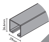
Aluminijska vodilica 2m, 3m, 4m
