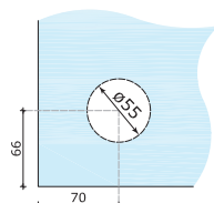
Brava podna s cilindrom i prihvatnikom 70x115 mm, inox SAT
