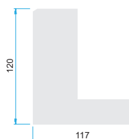
Završna kapica profila IG OG M50-ZM
