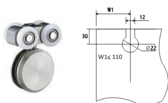
Nosač stakla
