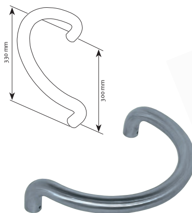
Rukohvat dužina 330 mm promjer Ø32 priprema stakla Ø16 mm u paru
