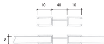
Brtva dupla 3000 mm, za staklo 8 mm FK MZ301BM-08
