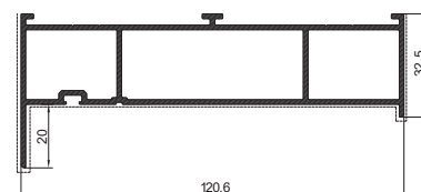
Bočni profil
