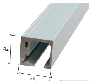
Aluminijska vodilica
