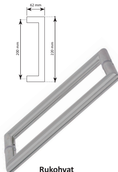
Rukohvat dužina 220 mm promjer Ø20 priprema stakla Ø12 mm u paru
