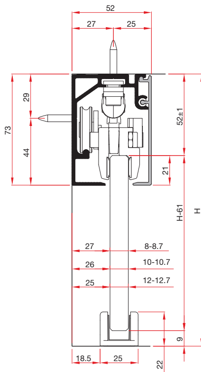
Vodilica
