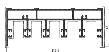
Gornji profil
