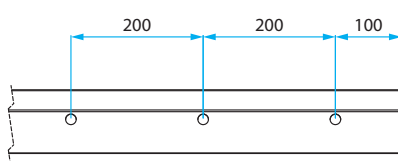
raspored rupa za fiksiranje stakla
