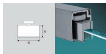
Kotač gornje vodilice
