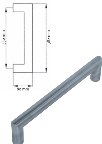
Rukohvat dužina 382 mm promjer Ø32 priprema stakla Ø16 mm u paru
