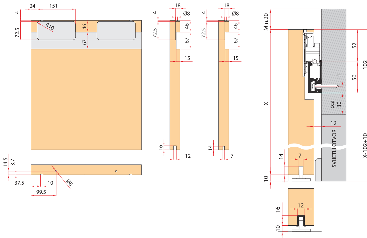
Podni profil 1X
