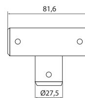
T konektor* šipka-šipka
