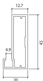
Alu profil za staklo debljina stakla 4 mm
