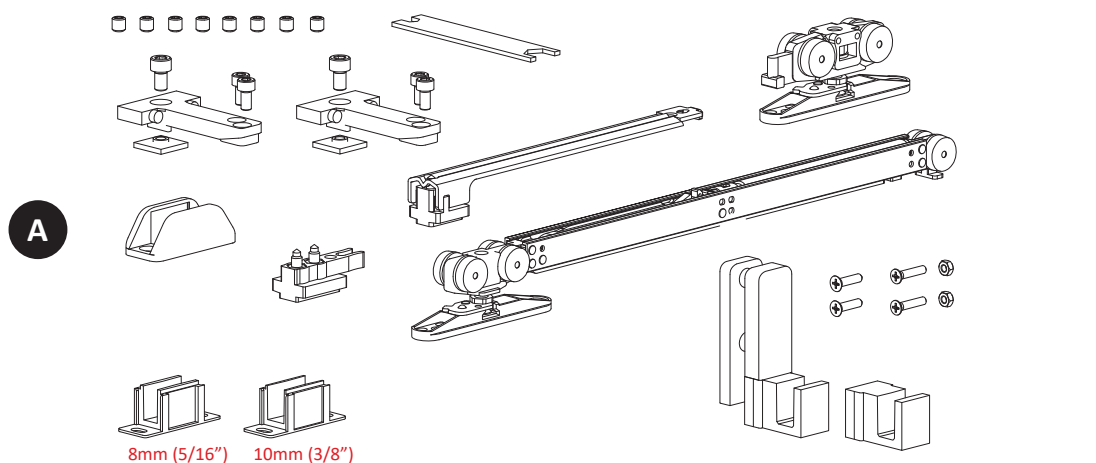
set za prvo krilo
