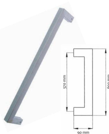
Rukohvat dužina 600 mm 30 x 30 mm priprema stakla Ø16 mm u paru
