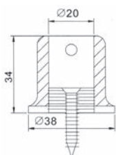
Konektor* zid-šipka
